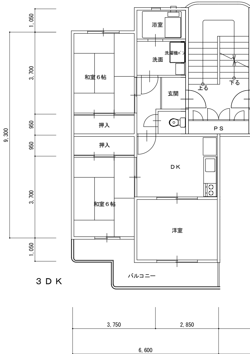
H 5 亀野住宅 A 棟平面図
