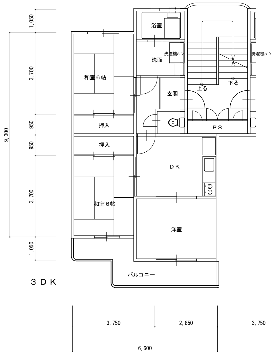
H 5 亀野住宅 B 棟平面図
